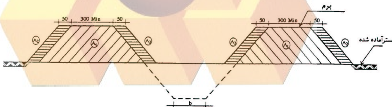
شکل ۴-۶. شمای مقطع خاکریزی
