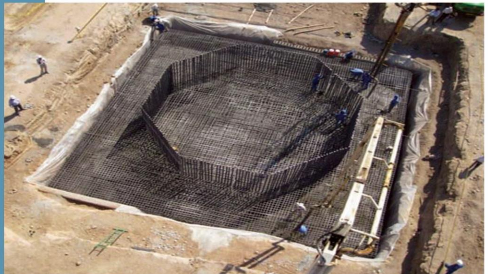
▶ اجرای آرماتور بندی فونداسیون تجهیزات (Vessel)
